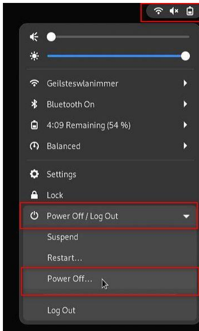
Abbildung 15: Power Off Menü – Auswahl Power Off
