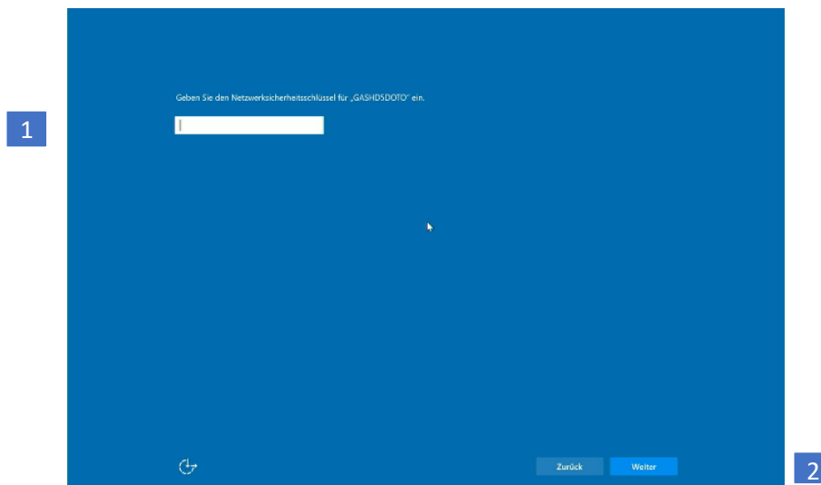
Abbildung 3: Netzwerksicherheitsschlüssel eingeben
