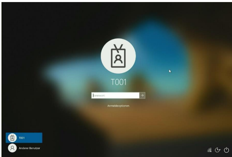
Abbildung 7: Anmeldebildschirm
